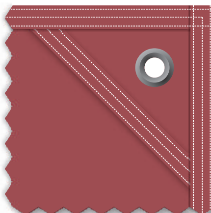
OX - 04 , trīskāršā vīle ar iestiprinātu kniedi
