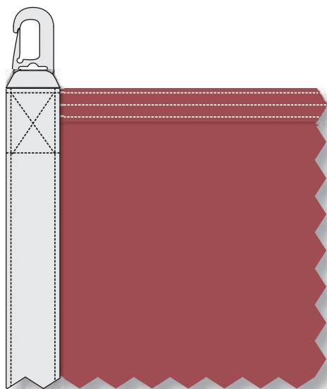
OX - 02 , lente ar karabīni no augšpusēs
