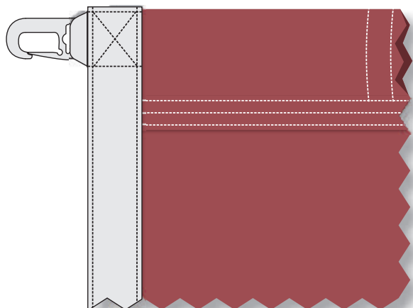
OX - 04 , lente ar karabīni un kabatu (Banner Bar)
