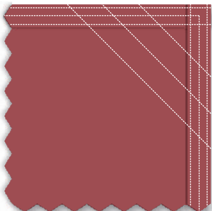
OX - 11 , trīskāršā vīle ar apšuvumu stūru nostiprināšanai
