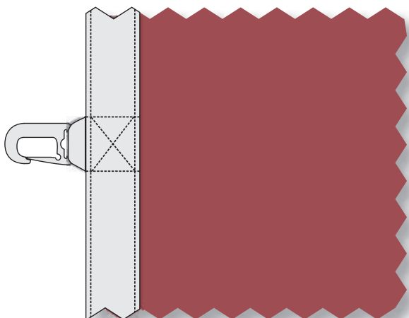
OX - 03 , lente ar karabīni no sāna
